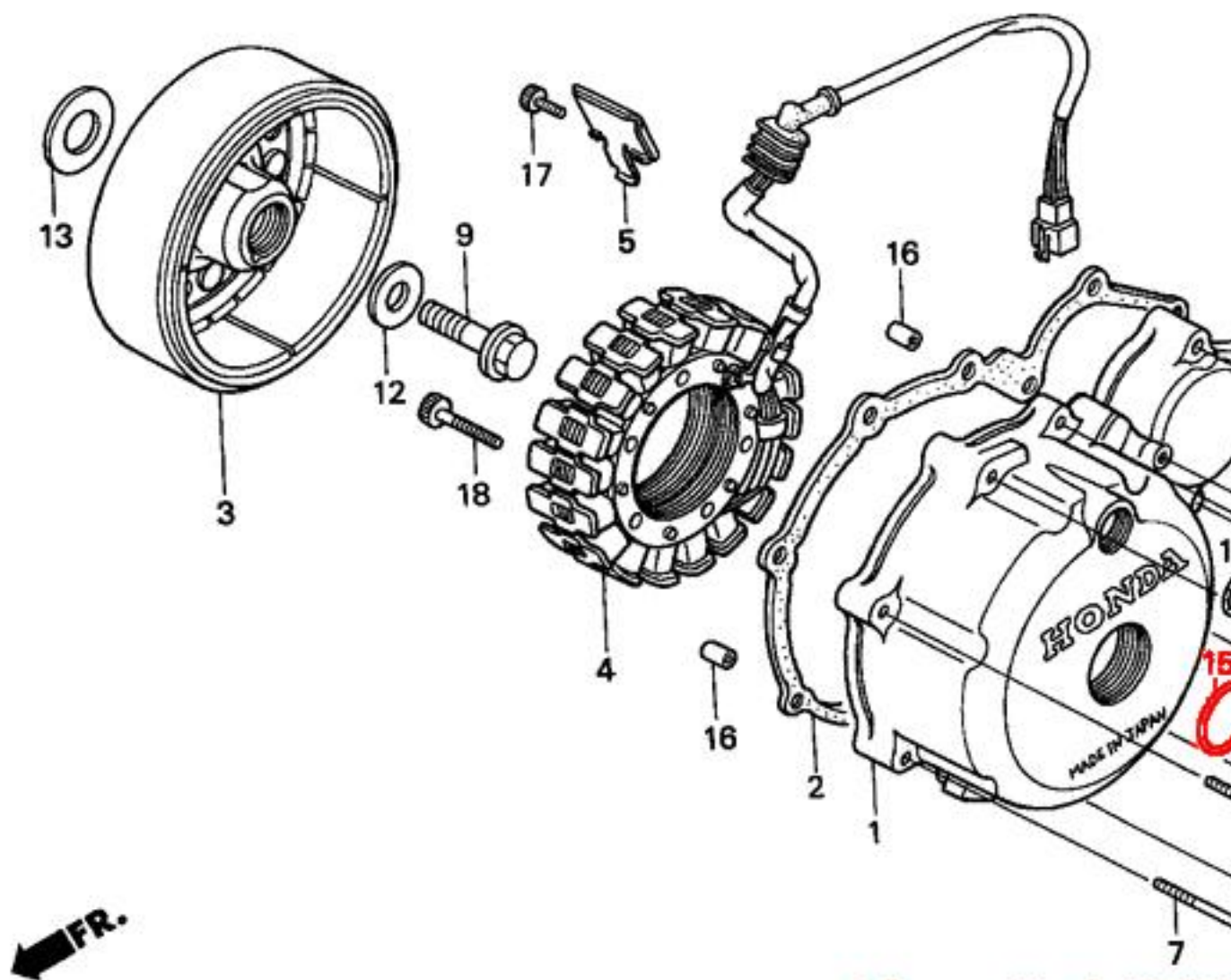
Schemat: Honda XL600V
